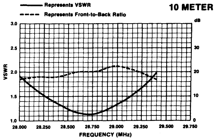
VSWR/Front-to-Back Charts
